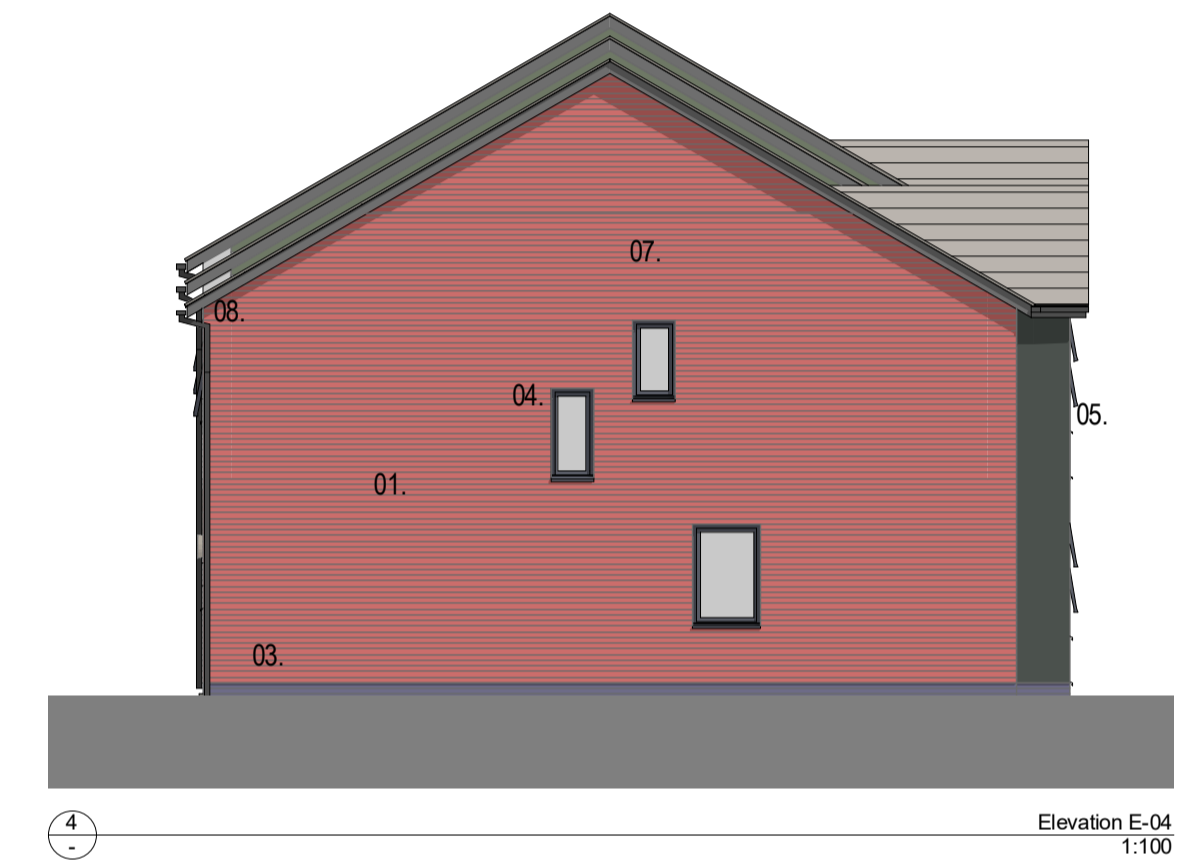
Elevation E-04 1:100
