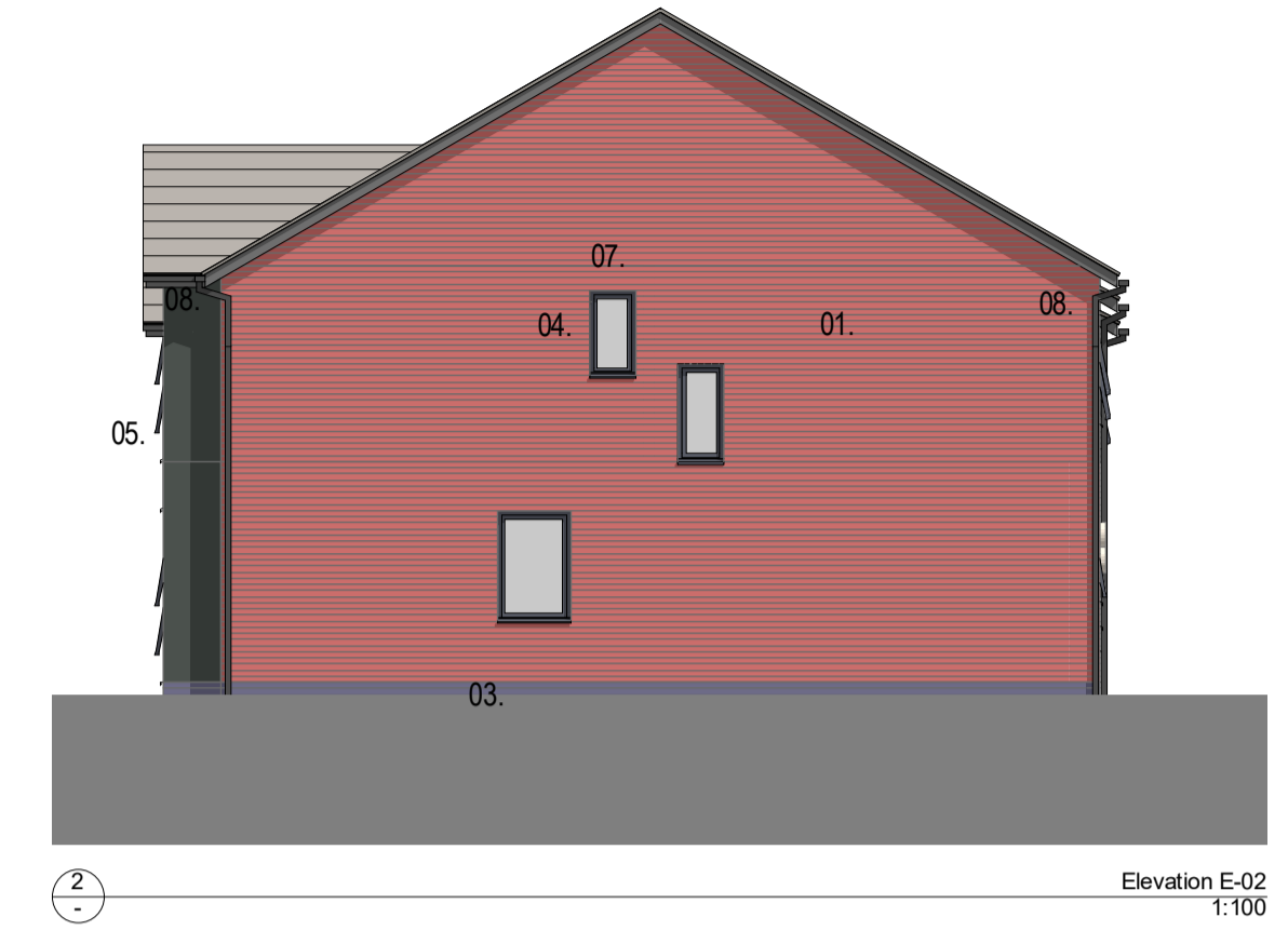
Elevation E-02 1:100
