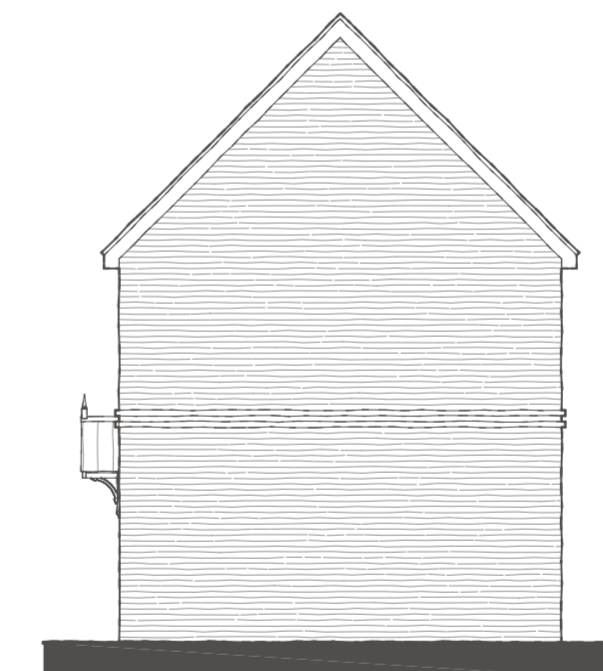
Elevation B
